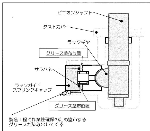
ピニオンシャフト部の断面図
